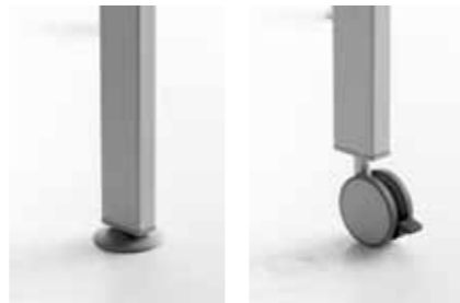
Nivelador y ruedas con freno Niveleur et roulettes freins Levellers and casters
